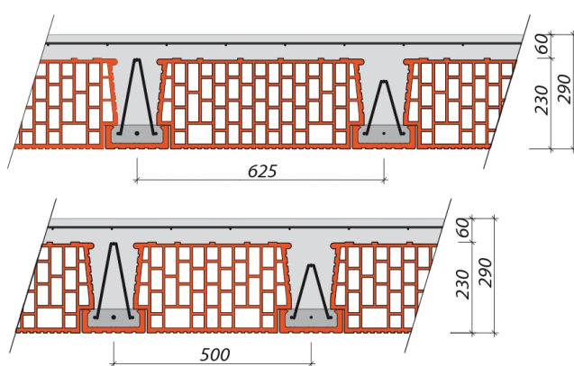
Deckendicke 290 mm
